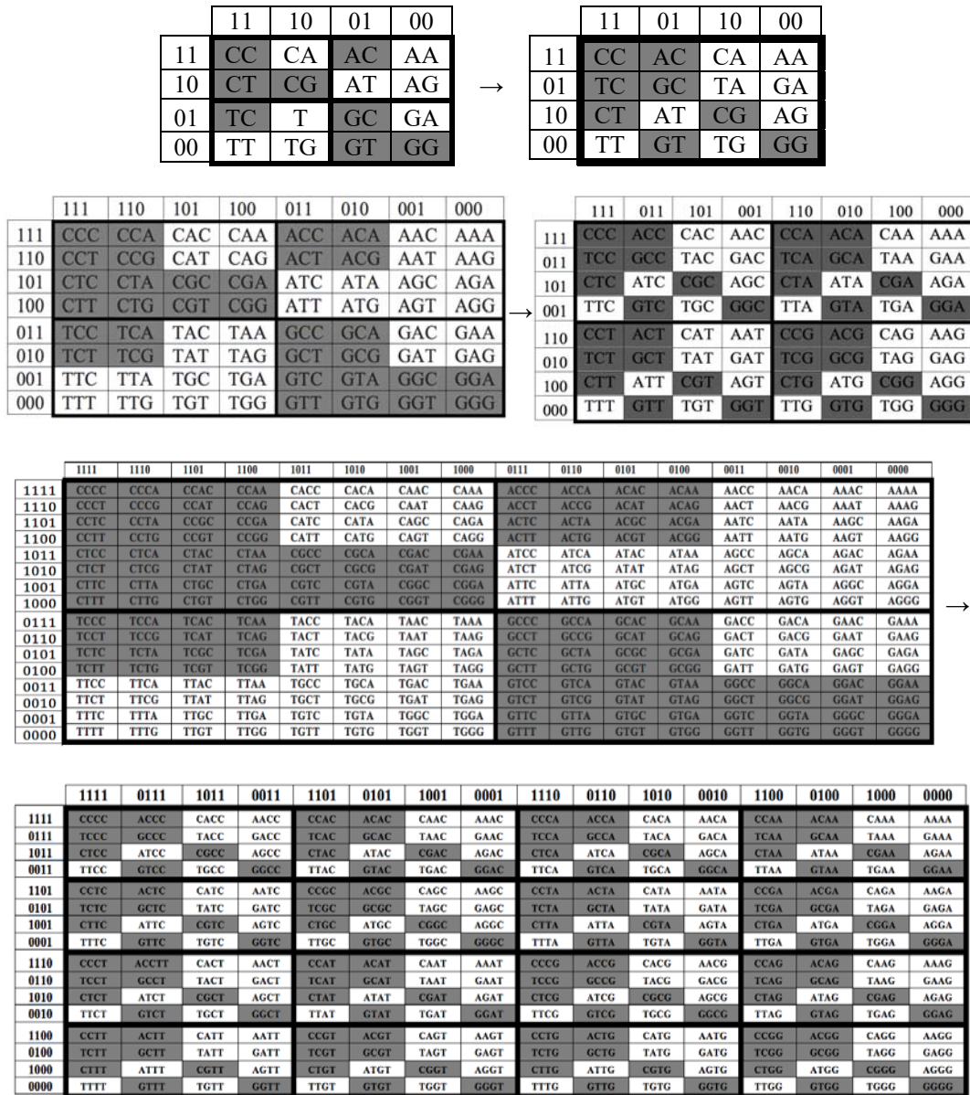
Рис. 5. Трансформация мозаичных алфавитных матриц [C, A; T, G]^{(n)} из рис. 4 в новые мозаичные алфавитные матрицы бит-реверсий в бинарных номерах столбцов и строк исходных матриц
