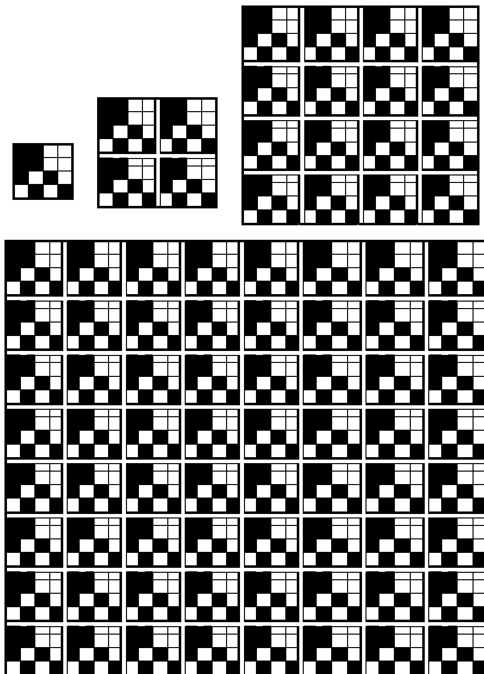
Рис. 6. Генетические «матричные кристаллы», представляющие в численной форме взаимно связанные мозаики символьных матриц [C, A; T, G]^{(n)} реверс алфавитов ДНК из рис. 5. Каждая черная клетка матриц содержит число +1, а каждая белая – число –1. Показанные многоблочные матрицы являются колониями или объединениями одной и той же (4 \times 4) -матрицы ( \alpha -матрицы), представляющей символьную матрицу [C, A; T, G]^{(2)} реверс алфавита 16 дуплетов
