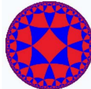
Рис. 7. Декомпозиция \alpha -матрицы на сумму 4 разреженных матриц ( \alpha = j_0 + j_1 + j_2 + j_3 ), набор которых замкнут относительно умножения и соответствует таблице умножения алгебры сплит-кватернионов Кокла. Дополнительно показан графический символ дисконной модели Пуанкаре гиперболической геометрии Лобачевского
