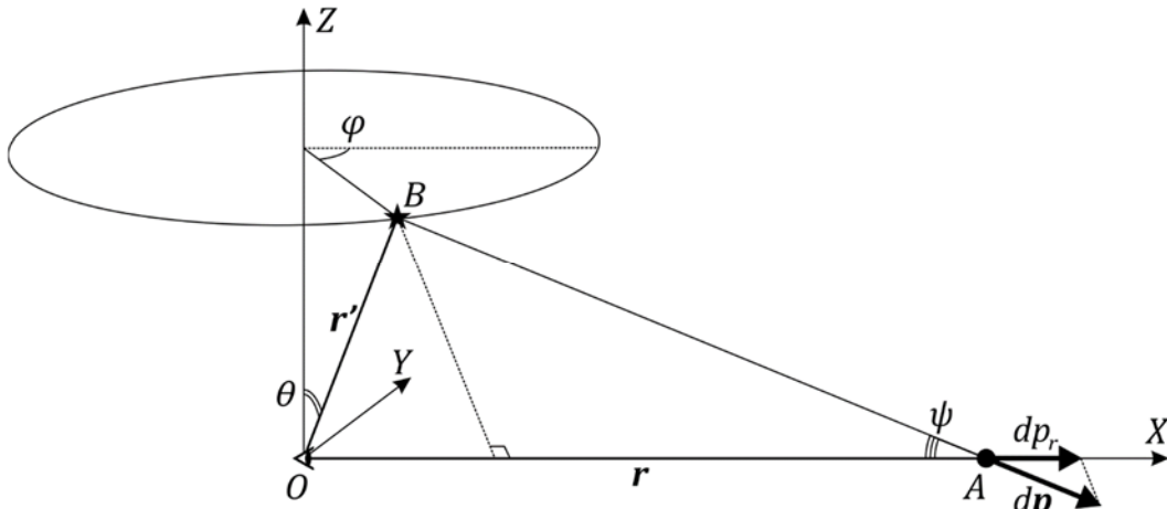
Рис. 1. Вклад излучателя в точке B в импульс поглотителя в точке A
